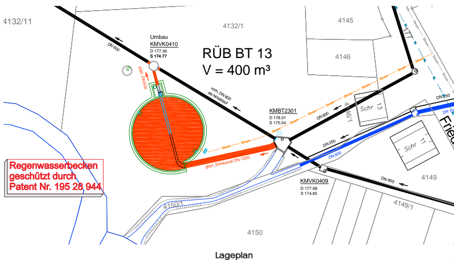
Lageplan
