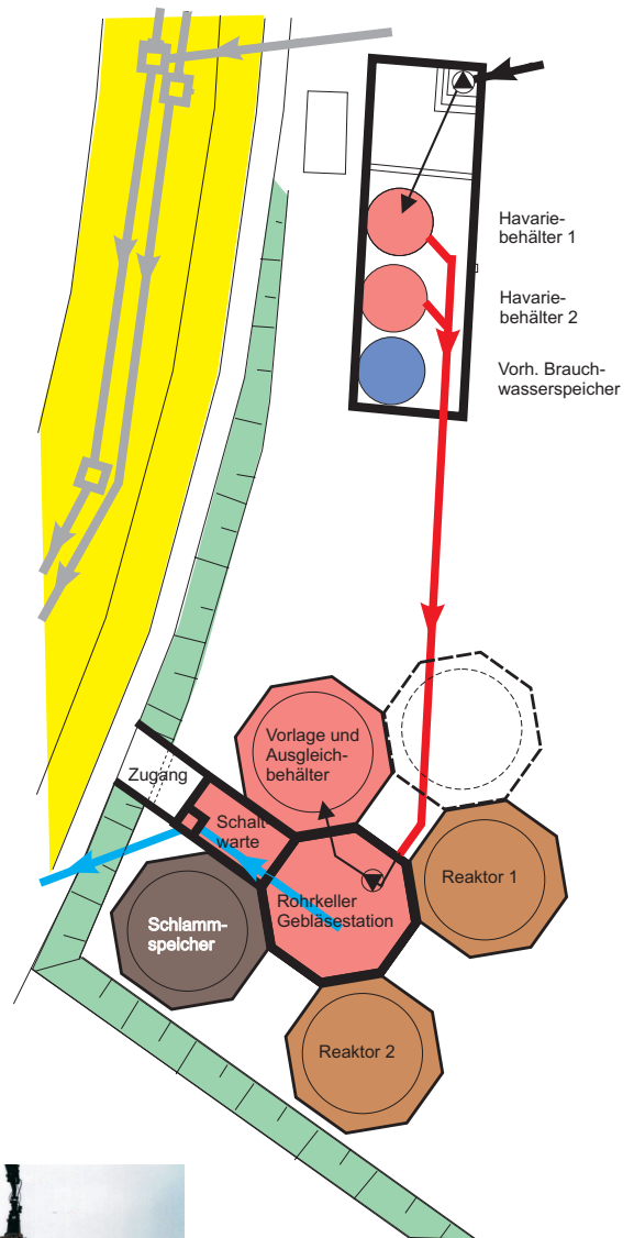
Lageplan
